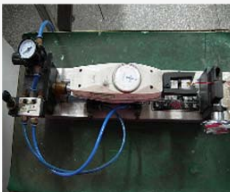
拉力計
